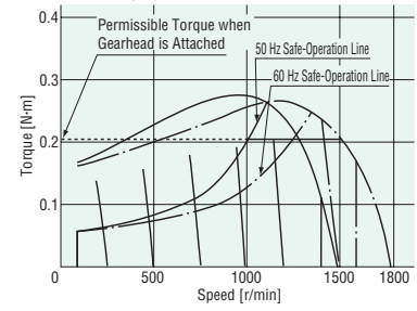
4IK25RGN(A)-CW2J/ES02
