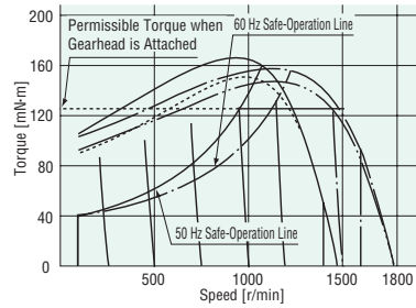
5IK60RGU(A)-CWE/ES02
