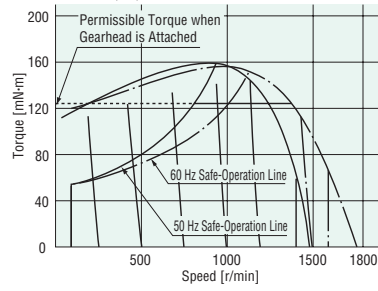
3IK15RGN(A)-CW2J/ES02
