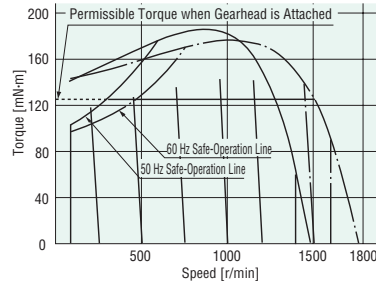
3RK15RGN(A)-CW2J/ES02
