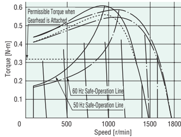
5RK40RGN(A)-CW2E/ES02
