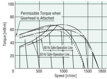
5IK40RGN(A)-CW2E/ES02
